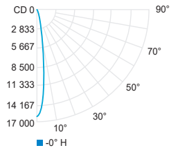
Spot 13° (3000K, 92CRI)
