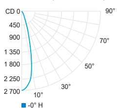
Flood 27° (3000K, 90CRI)
