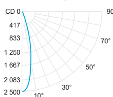
Medium 24° (3000K, 90CRI)
