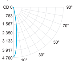
Spot 16° (3000K, 90CRI)
