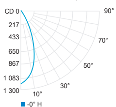
Wide flood 41° (3000K, 90CRI)
